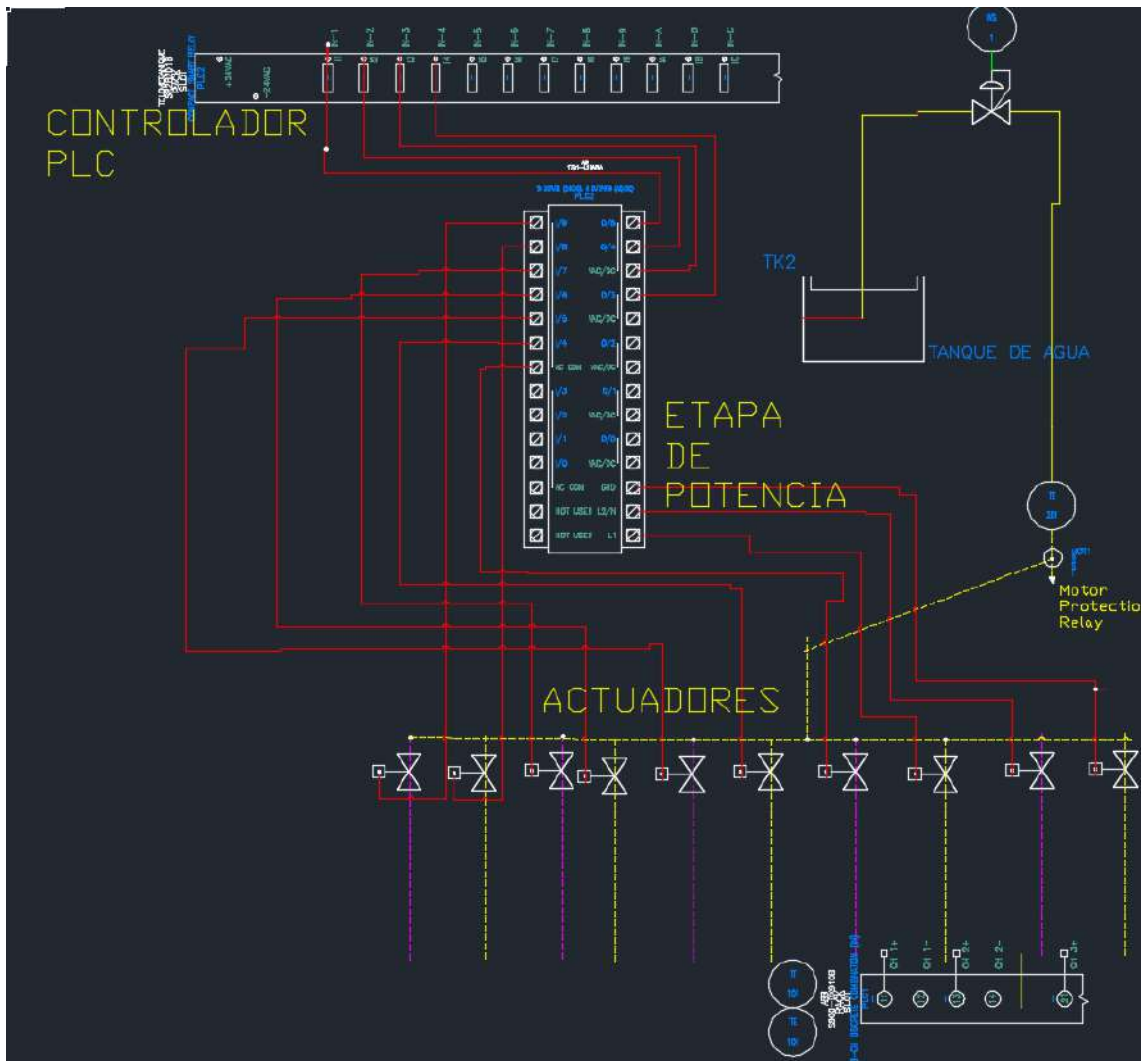
Figura 11-2: Diagrama de etapas de Control
