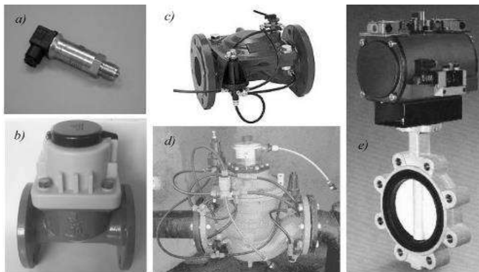
Figura 6-1. Sensores y actuadores; transductor de presión (a), contador de pulsos (b), electroválvula (c), válvula pilotada (d) y de mariposa motorizada (e) Fuente: (Ruiz Canales & Molina Martinez, 2011).
