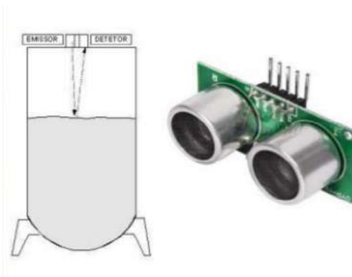
Figura 8-1. Sensor de nivel continuo (Ultrasónico)
