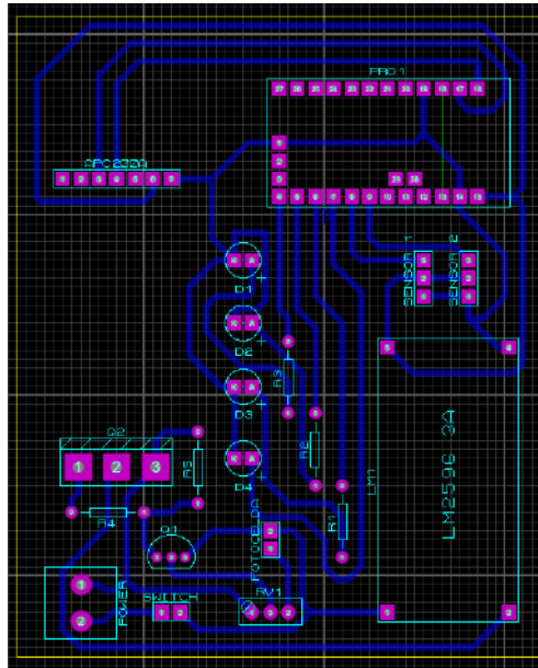
Figura 6-2. PCB Layout placa transmisora Fuente: Kleber Chulde 2017.
